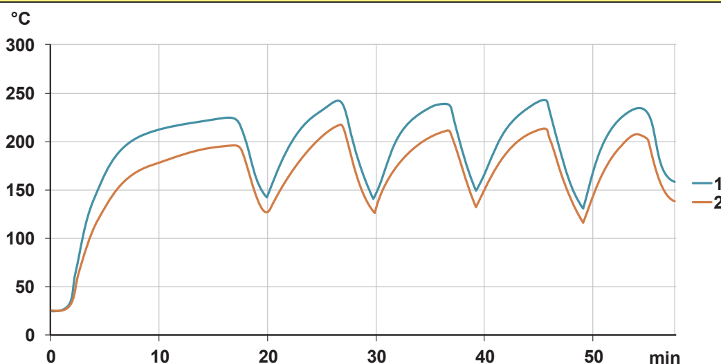
Misurazione della temperatura effettuata su un nastro di silicone di 200mm di larghezza montato su un fusto da 55 galloni (200 litri). Potenza 2250W (0.75W/cm 2 ), controller PID con sensore posizionato al centro del serbatoio vuoto. Temperatura superficiale limitata a 190°C da un termostato a disco.
